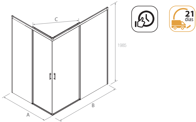
ANGULAR DE DUCHA
