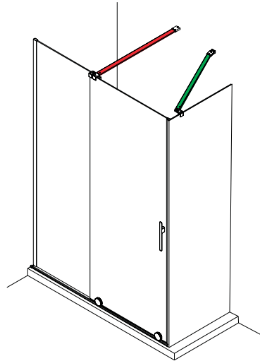
Mampara angular (pag 456) compuesto por un frontal, con tensor frontal, con lateral fijo y kit magnético angular.
