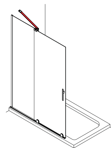
Mampara frontal (pag 454) compuesto por tensor angular
