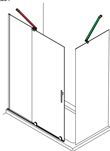
Mampara angular (pag 456) compuesto por un frontal, con tensor angular y con lateral fijo.
